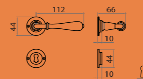
3 Ros 45x10 V.V. Mont. n°107
