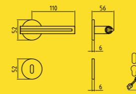
1 Ros 52x6 Mont. n°103-104
