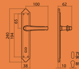
1 Placca LADY Mont. n°41
