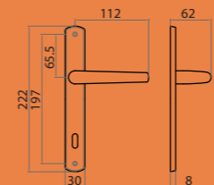
2 Placca STRETTA Mont. n°37
