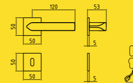
1 Ros 50x50x5 (molla ambidestra - maniglia non solidale) Mont. n°66 - 67
