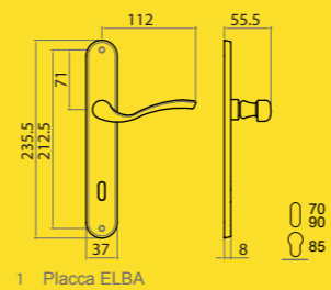
1 Placca ELBA Mont. n°35
