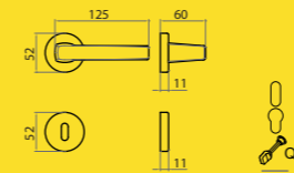
1 Ros 575 Mont. n°95-96
