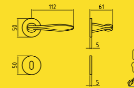
1 Ros ribassata (molla dx e sx - maniglia non solidale) Mont. n°91-92
