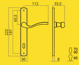
2 Placca STRETTA Mont. n°37
