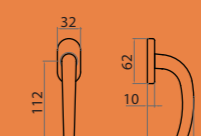
6 DK-2P Mont. n°8
