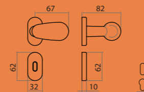
2 Ros 0006 Mont. n°25
