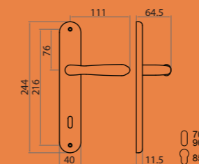
1 Placca UNO Mont. n°36
