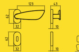
2 Ros 0006 Mont. n°20
