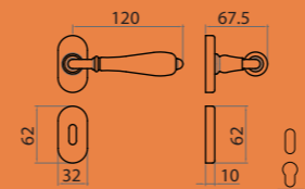
2 Ros 0006 Mont. n°25
