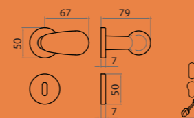
1 Ros 0005 Mont. n°93-94
