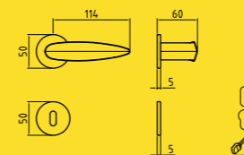
1 Ros ribassata (molla dx e sx - maniglia non solidale)
