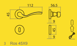
3 Ros 45X9 Mont. n°88-89
