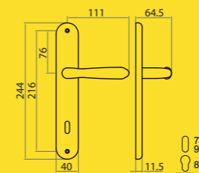
1 Placca UNO Mont. n°36
