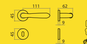
3 Ros 45X9 Mont. n°88-89
