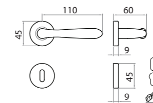
1 Ros 45x9 Mont. n°88-89
