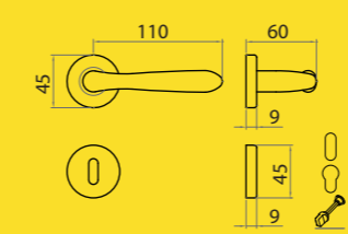
1 Ros 45x9 Mont. n°88-89
