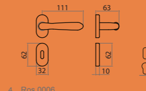
4 Ros 0006 Mont. n°25
